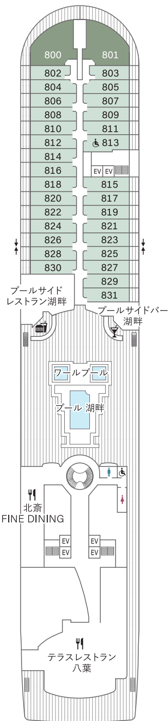
デッキ8 [DECK 8]
